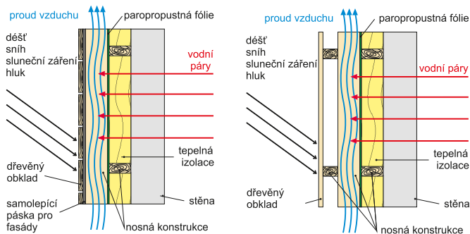
Schéma konstrukce opláštěné horizontálně orientovaným obkladem
